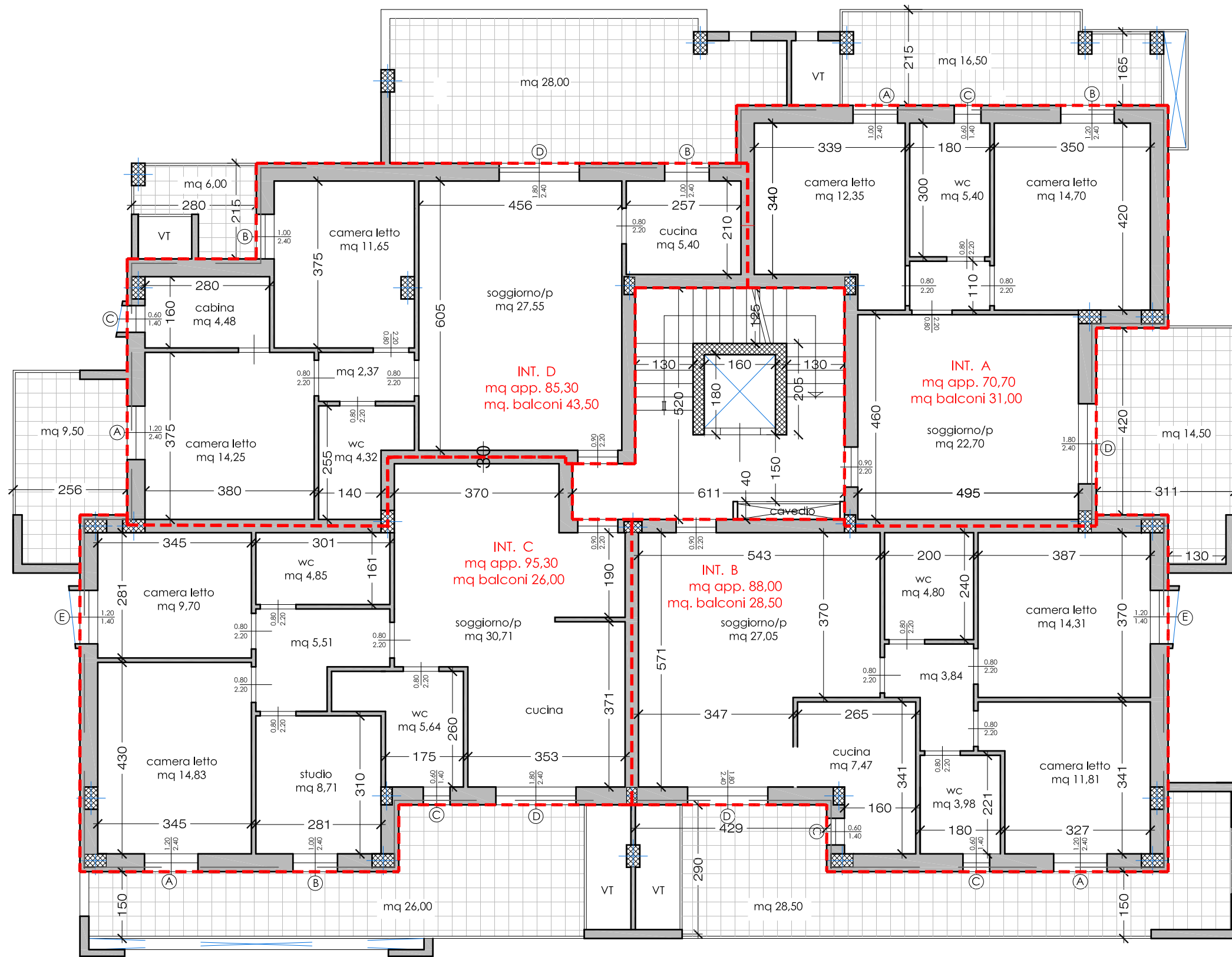
Pianta piano SECONDO - scala 1:100
