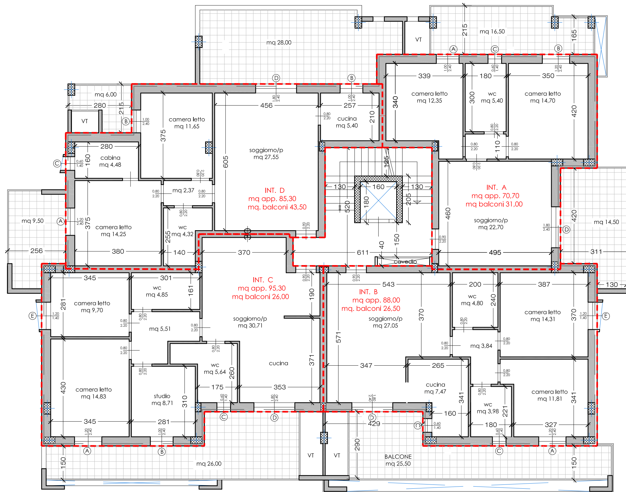
Pianta piano QUINTO - scala 1:100
