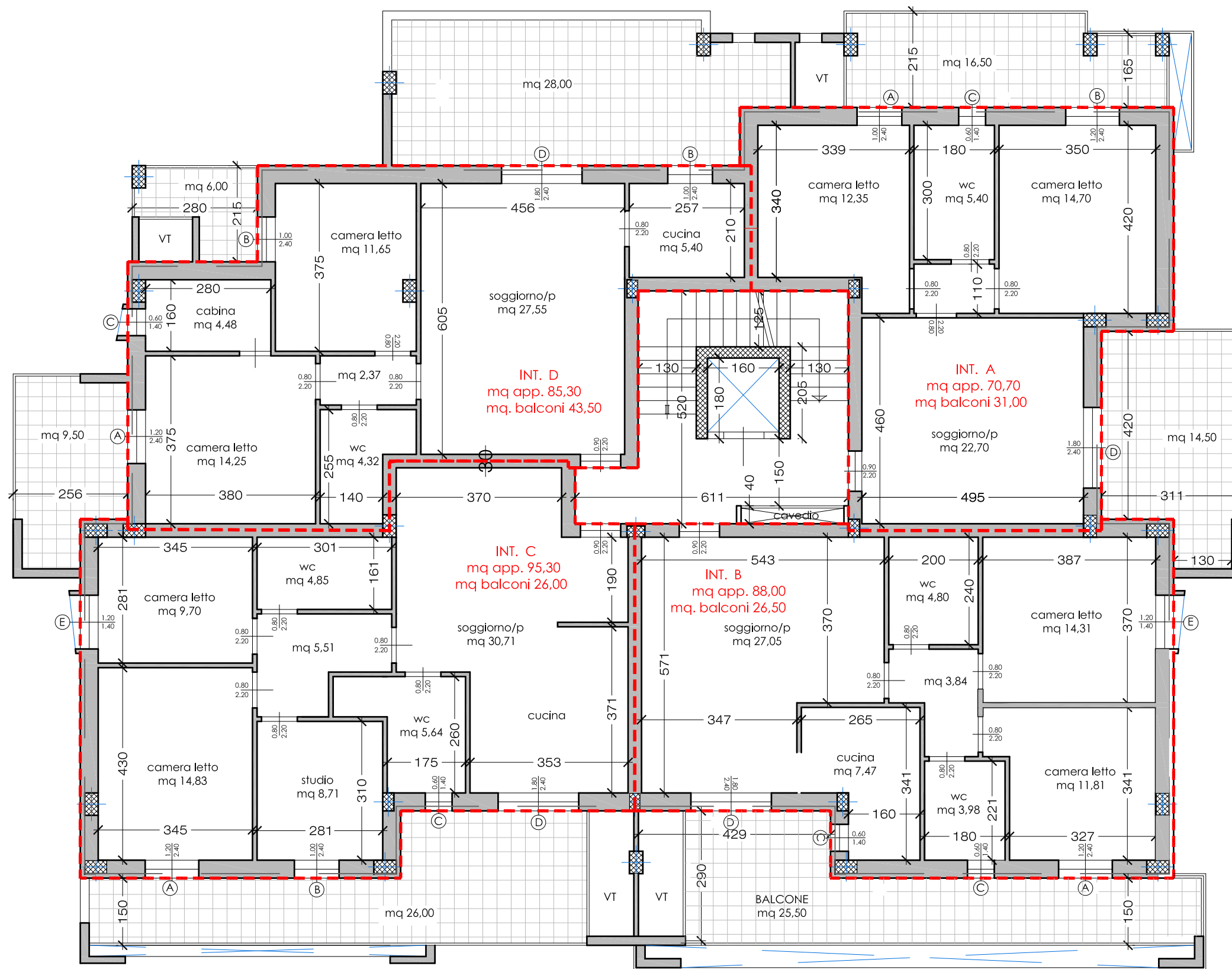
Pianta piano SESTO - scala 1:100
